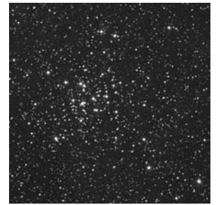
M36
