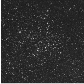
M38
