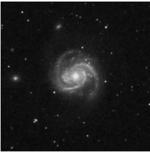
M100
