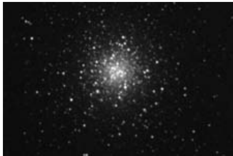
M53
