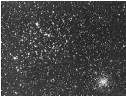
M35 & Ngc2158
