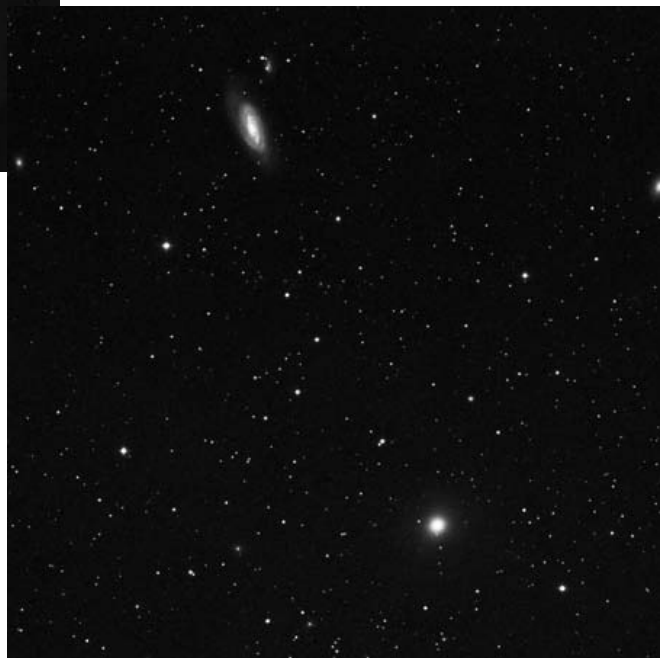
M89 & M90
