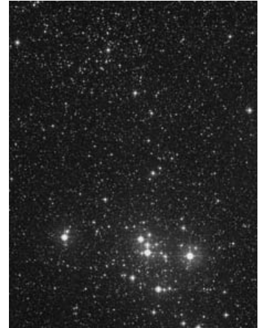
M47
