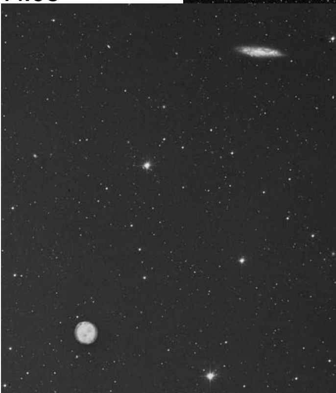
M97 & M105
