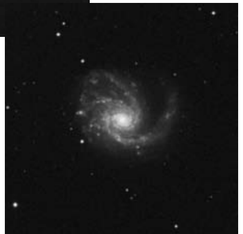
M99
