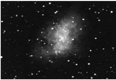
M1
